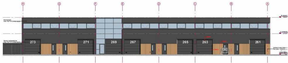
1 Noord-oostgevel schaal 1:100
